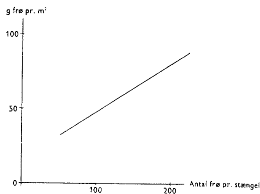
Fig. 2. Korrelation mellem frøudbytte (y-aksen) og antal frø pr. stængel (x-aksen), r=0,5887^{***} , y=16+0,3217x , n=288 , \bar{y}=56 g frø pr. m^2 , \bar{x}=123 frø pr. stængel.
