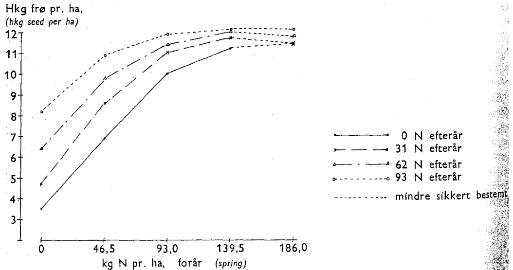
Fig. 1. Udbyttekurver for stigende mængder forårsudbragt N ved 0, 31, 62 og 93 kg N udbragt om efteråret. (Yieldcurve for increasing quantities N as spring dressing at autumn dressings of 0, 31, 62 and 93 kg N).
