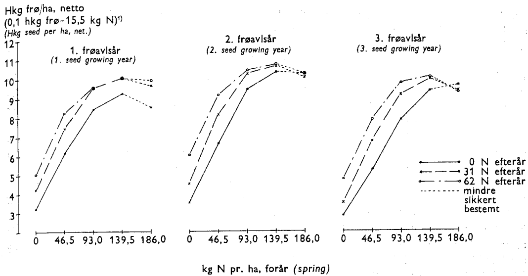
Fig. 2. Udbyttekurver for stigende mængder forårsudbragt kvælstof ved 0, 31 og 62 kg N udbragt om efteråret. (Yieldcurve for increasing quantities nitrogen as spring dressing at autumn dressings of 0, 31 and 62 kg N).
