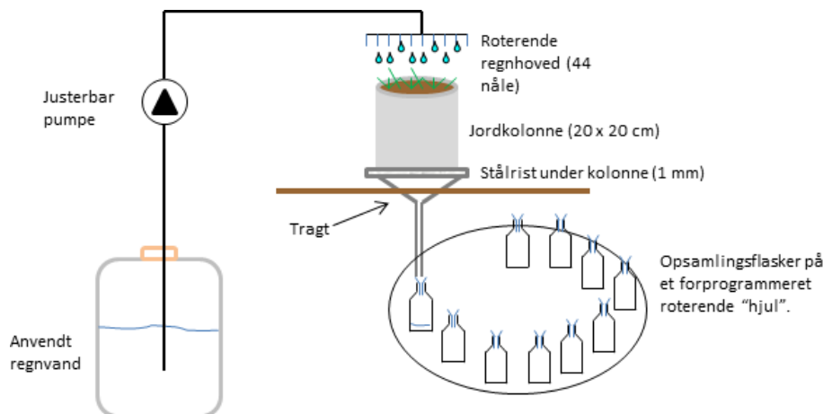
Figur 1. Forsøgsopstilling
